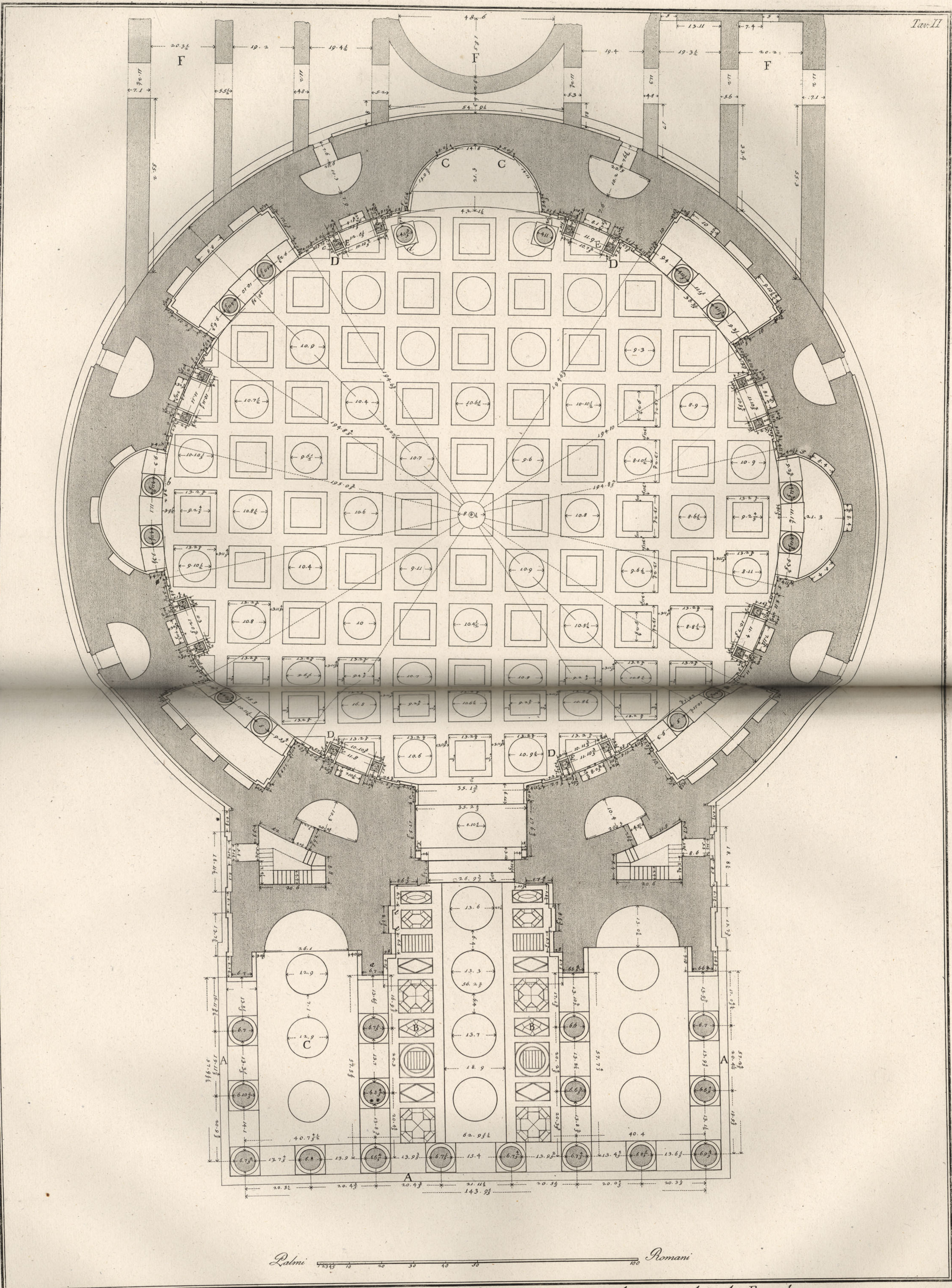
Ichnografia dello stato presente del Pantheon di Marco Agrippa ora volgarmente detto la Rotonda A. Gradi moderni intorno del Pronao o Portico B. Nuovo pavimento di mattoni in cortello. C. Pilastri moderni che adornano l'altare maggiore. Li piedestalli dell' Edicole. D. sono stati interrotti in E. volando la cimasa per introdurre le mense degli altari F. Avanzi delle Terme di Agrippa. Car. Fra. I. Traversari delinea ed incisit
