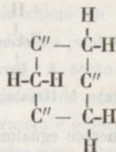
Benzina ( \alpha )
