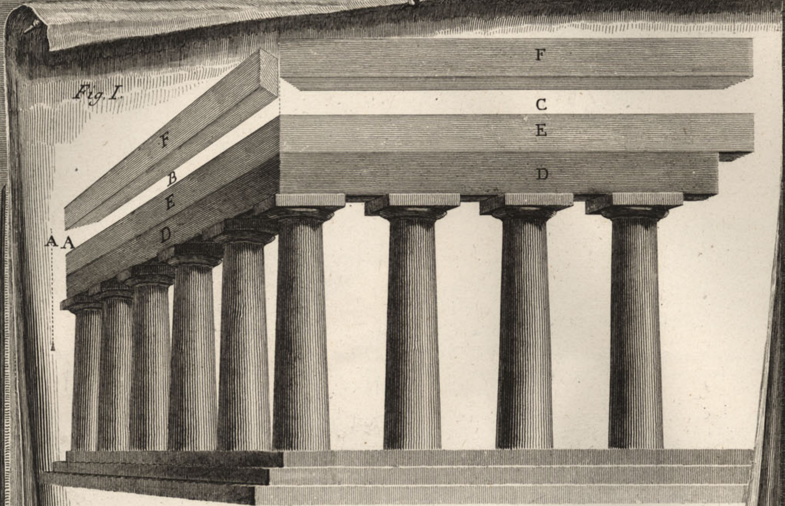
A. Directio. B. Frons. C. Latus. D. Epistylia. E. Tigna. F. Demonstratio compactionis angularis eorumdem tignorum
