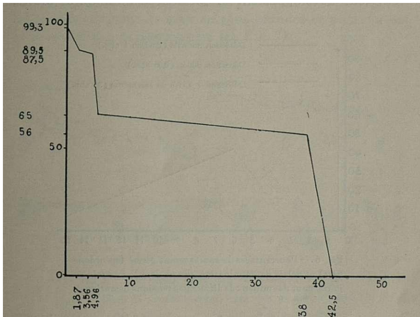
Fig. 5. — Pourcentage de spores ayant germé (en ordonnées) en fonction de la tension osmotique du milieu de culture (en abscisses) pour les milieux concentrés.
