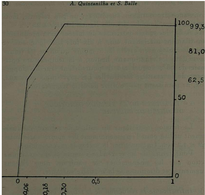
Fig. 4.—Pourcentage de spores ayant germé (en ordonnées) en fonction de la tension osmotique, mesurée en atmosphères, du milieu de culture (en abscisses) pour les milieux dilués.
