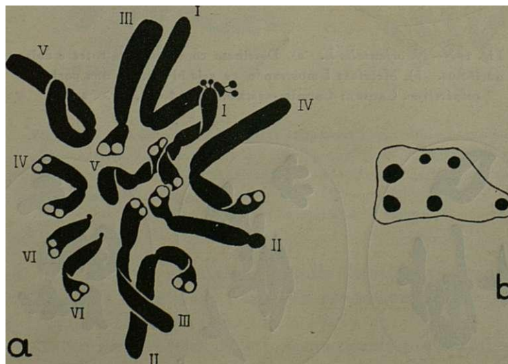
Fig. 16.— N. ciliaris DC. a), Placa ecuatorial numa célula do meristema radicular mostrando os seis pares de cromosomas existentes. Navachine; Violeta de genciana. X 2.700. b), Núcleo de uma telofase precoce mostrando seis nucléolos. Altmann. X 2.700.
