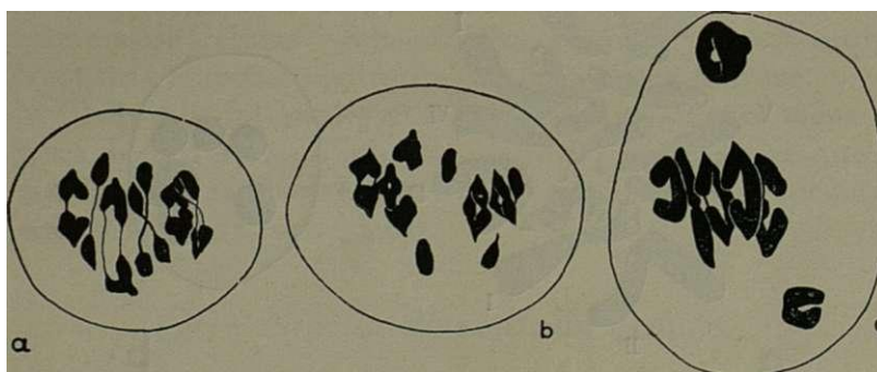
Fig. 33. — N. diversifolia Franch. a), Metáfase I mostrando os sete bivalentes. b), Metáfase I em que três dos bivalentes se encontram divididos. c), Metáfase I mostrando dois bivalentes fora do plano equatorial. Carnoy; Carmím-acético. a e b, \times 1.600 ; c, \times 2.700 .
