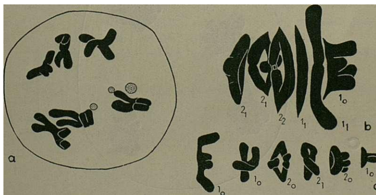
Fig. 23.— N. arvensis L. a), Diacinese mostrando os seis bivalentes e três nucléolos. b), Metafase I com os seis bivalentes nas posições respectivas. c), Metafase I em que os bivalentes foram desenhados separadamente. Carnoy; Carmim-acético. X 2.700.
