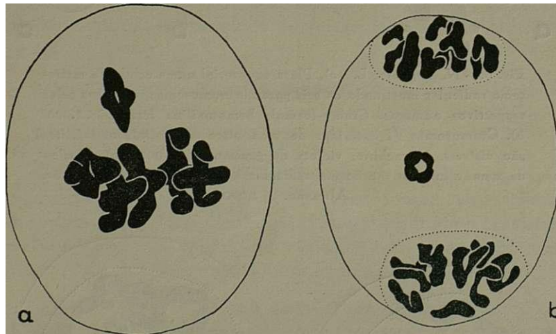
Fig. 8.— N. ispanica L. a), Metafase I com um bivalente fora do plano equatorial. b), Telofase I mostrando um bivalente que permaneceu no plano equatorial. Carnoy; Carmim-acético. X 2.500.
