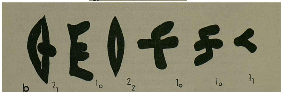
Fig. 30. — N. Nigellastrum (L.) Willk. a), Diacinese com seis bivalentes e um nucléolo. Carnoy; Carmim-acético. \times 1.600 . b), Metafase I em ue os bivalentes foram desenhados separadamente. Carnoy; Carmim-acético. \times 2.700 .
