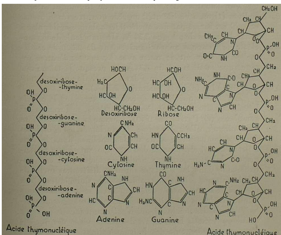
Fig. 4.—Formules de l'acide thymonucléique et de ses constituants.
