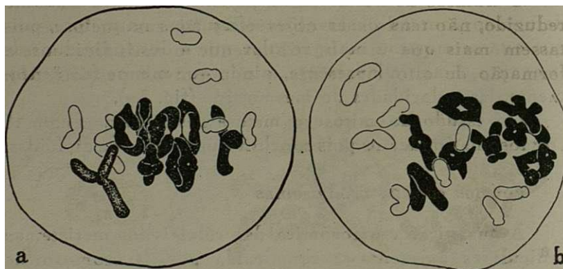
Fig. 6. — Ranunculus Ficaria L. (n.º 130). a, Metafase da divisão I mostrando um trivalente, sete bivalentes e sete univalentes. b, Idem com oito bivalentes e oito univalentes. Álcool acético; carmim-acético. X 1100.
