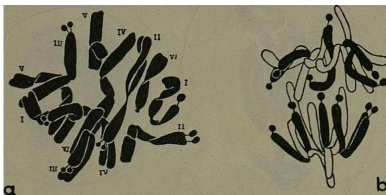
Fig.13.— N. orientalis L. a), Placa equatorial numa célula do meristema radicular; os seis tipos de cromosomas estão indicados pelos respectivos números. b), Anafase mostrando em cada metade os seis cromosomas compridos — tipos I, II e III — providos de satélite. Cromo-formol; violeta de genciana. \times 2.000 .
