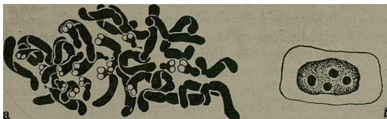
Fig. 8. — Ranunculus Ficaria L. (n.º 143). a, Placa equatorial numa célula do meristema radicular. Navachine; violeta de genciana \times 2330 . b, Núcleo em repouso mostrando 4 nucléolos. Flemming; violeta de genciana. X 1800.
