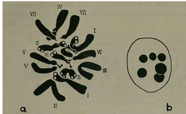
Fig. 31.— N. N. Franch. a), Placa equatorial numa célula do meristema radicular. Vêem-se os 7 tipos de cromosomas. Nava-chine; Violeta de genciana. X 2.700. b), Núcleo de uma célula do meristema radicular mostrando seis nucléolos. Altmann. X 2.700.
