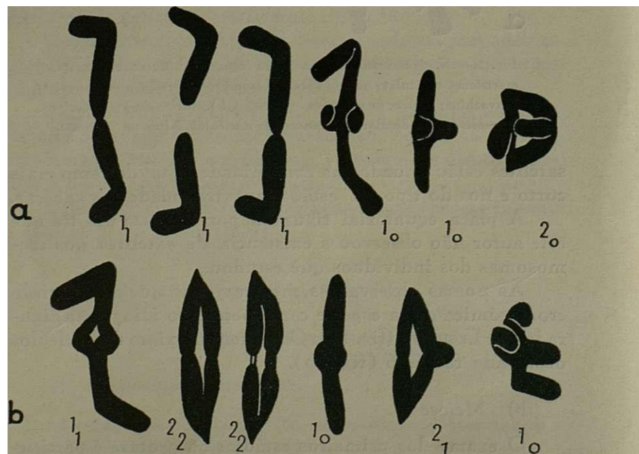
Fig. 3.— N. damascena L. Bivalentes de duas metafases desenhados separadamente. Carnoy; Carmim-acético. \times 2.000 .
