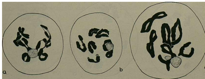
Fig. 32.— N. N. Franch. a), Diacinese com um nucléolo em relação com os três bivalentes nucleolares. b), Diacinese com dois bivalentes ligados a um nucléolo e um outro tendo um pequeno nucléolo ligado a cada um dos cromosomas. Notam-se em três dos bivalentes regiões que coram menos intensamente. c), Diacinese com um nucléolo estrangulado, tendo ligados dois bivalentes. Carnoy; Carmim-acético. a e b, X 1.600. c, X 2.700.
