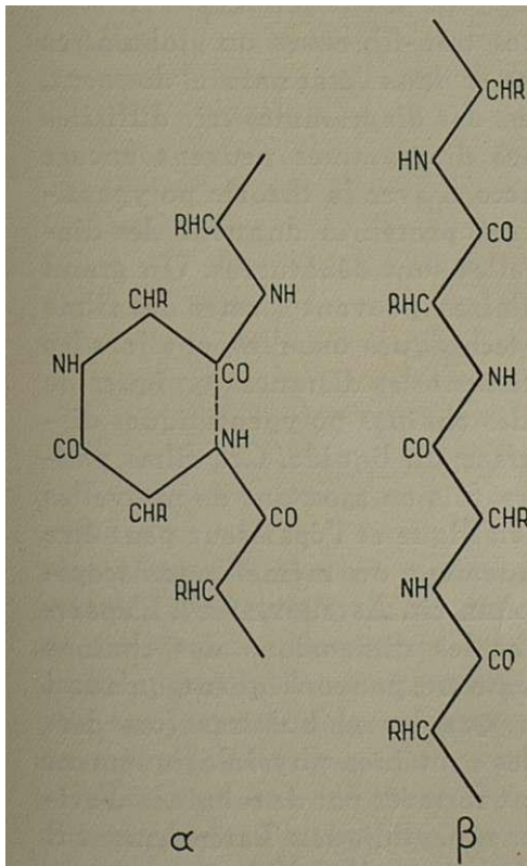
Fig. 1.—Les deux formules de la kératine. — radicaux des acides aminés; \alpha — forme contracté normale; — forme distendue.
