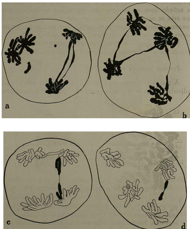
Fig. 4. — Ranunculus Ficaria L. (n.º 150). a, Anafase II mostrando duas pontes devidas a «loop-chromatids», um fragmento e um univalente. b, Anafase II com 4 pontes, duas persistentes da primeira divisão e duas formadas na segunda. c, Anafase II em que se vê uma pseudo-ponte. d, Divisão de um univalente mostrando coalescência entre os topos dos cromatídios. Álcool acético; orceina acética. X 1100.
