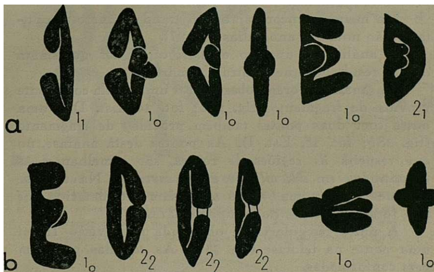
Fig. 27. — N. gallica Jord. — Duas metafases I em que os bivalentes foram desenfiados separadamente. Carnoy; Carmim-acético. X 2.700.
