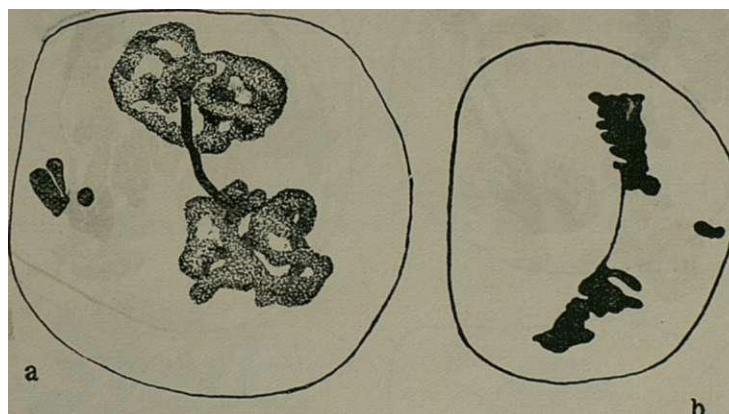
Fig. 3.— Ranunculus Ficaria L. a (n.º 163), Telofase I mostrando uma ponte, um fragmento e um univalente. X 1800. b (n.º 150), Ponte persistindo da primeira divisão e unindo as placas da divisão II. À direita um univalente. Álcool acético;orceína acética. X670.
