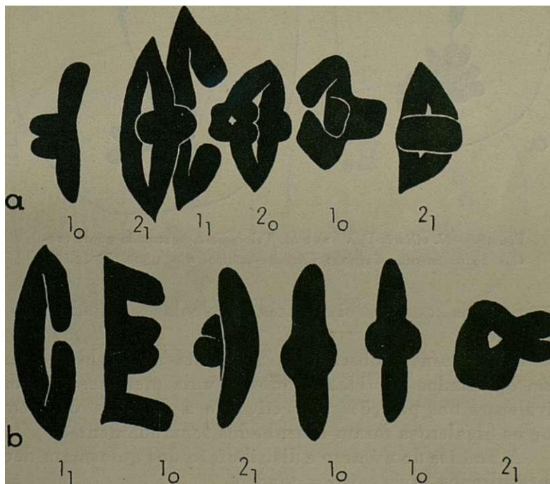
Fig. 18. — N. ciliaris DC. a), Metafase I com os seis bivalentes nas posições respectivas. b), Metafase I em que os bivalentes foram desenhados separadamente. Carnoy; Carmim-acético. X 2.700.
