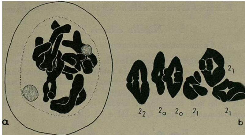
Fig. 14.— N. orientalis L. a), Diacinese com seis bivalentes e dois nucléolos. b), Metafase I mostrando os seis bivalentes nas posições respectivas. Carnoy; Carmim-acético. a, X 2.000, b, >2.500,
