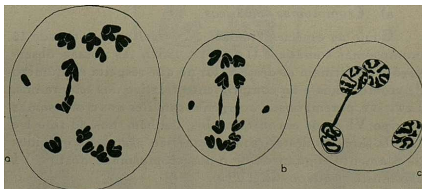
Fig. 28. — N. gallica Jord. a), Anafase I com ponte provida de fragmento. b), Anafase I mostrando duas pontes com fragmentos. Carnoy; Carmim-acético. X 2.700. c), Telofase II com uma ponte. Carnoy; Carmim-acético. X 1.600.
