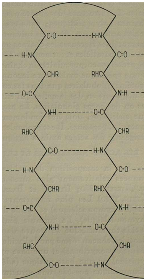
Fig. 3.— Représentation schématique du plie- ment d'une protéine globulaire. On remarque le rôle capital des liaisons H.
