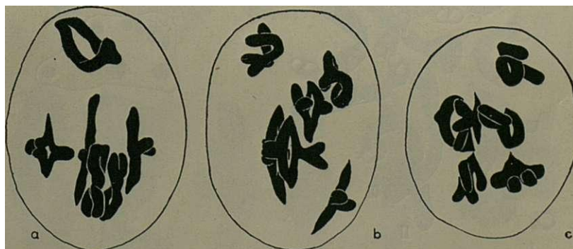
Fig. 15.— N. orientalis L. a), Metafase I com cinco bivalentes no plano equatorial e um na região de um dos polos. b) e c), Metafases I mostrando a não orientação de alguns dos bivalentes. Carnoy; Carmim-acético. X 2.500.
