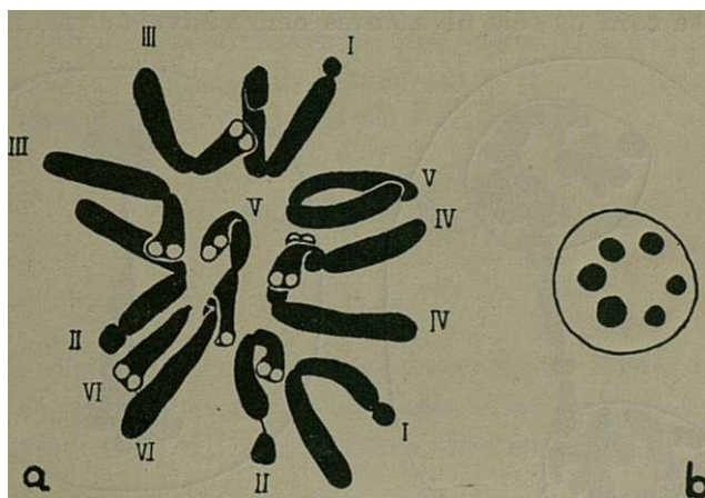
Fig. 22.— N. arvensis L. a), Placa equatorial numa célula do meristema radicular; vêem-se os seis pares de cromosomas com os respectivos números. Navachine; Violeta de genciana. X 3.700. b), Núcleo de uma célula do meristema radicular mostrando seis nucléolos. Altmann. X 2.700.
