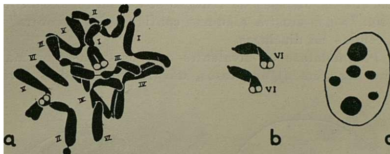
Fig. 6.— N. hispanica L. a), Placa equatorial numa célula do meristema radicular mostrando os seis pares de cromosomas indicados pelos respectivos números. Cromo-formol hematoxilina férrica. X 2.000. b), Cromosomas VI extraídos de uma placa equatorial; os satélites são visíveis. Navachine; violeta de genciana. X 2.000. c), Núcleo de uma célula do meristema radicular apresentando seis nucléolos. Altmann. X 2.000.
