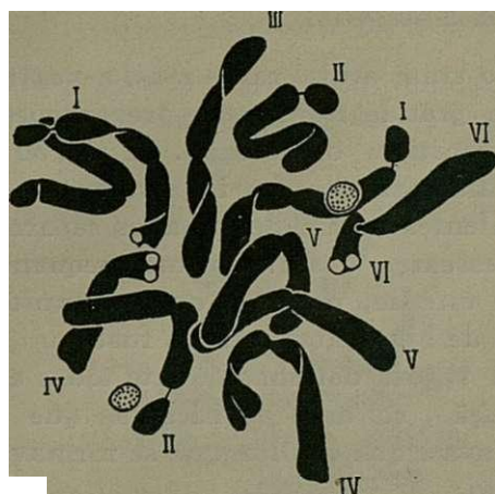
Fig. 29. — N. Nigellastrum (L.) Willk. a), Placa equatorial numa célula do vértice vegetativo da raiz, mostrando os seis tipos de cromosomas existentes. Vêem-se dois nucléolos que se não dissolveram. Navachine; Violeta de genciana. \times 2.700 . b), Telofase precoce mostrando seis nucléolos em cada um dos núcleos-filhos. Altmann. \times 2.700 .
