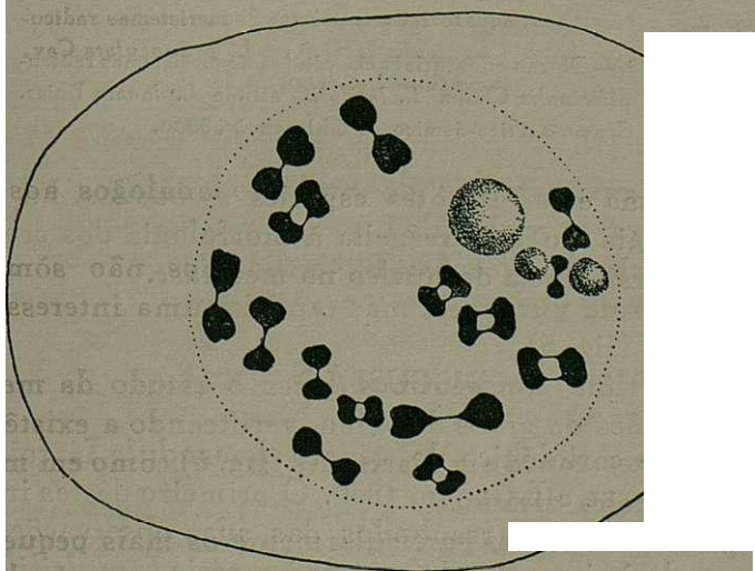
Fig. 6. — Dia cínese em uma célula-mãe de grãos de pólen d L. Stoechas L., forma albina. Álcool acético. X 1900.
