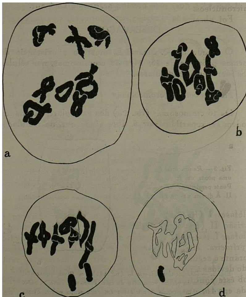
Fig. 2.— Ranunculus Ficaria L. (n.º 150). a , Diacinese com 8 bivalentes. b , Metafase I com 8 bivalentes. c e d , Metafase I com, respectivamente, 2 e 1 univalentes. Álcool acético;orceína acética. X 1280.
