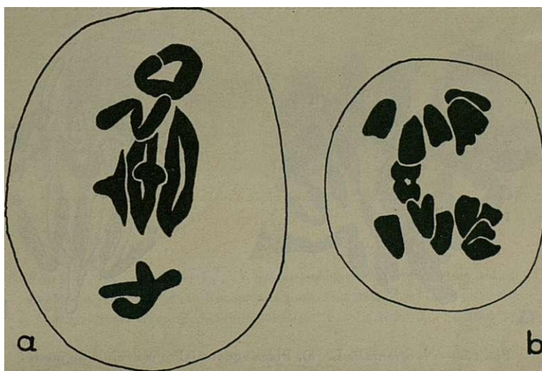
Fig. 12. — N. sativa L. a), Metafase I com três bivalentes no plano equatorial e três fora dele. b), Anafase I mostrando um bivalente que permaneceu no plano equatorial. Carnoy; Carmim-acético. X 1.600.
