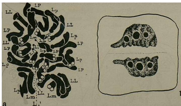
Fig. 5. — Ranunculus Ficaria L. a (n.º 130), Metafase numa célula do meristema radicular. Navachine; violeta de genciana. X 2330. b, Telofase numa célula do vértice vegetativo da raiz. Lewitsky; safranina verde luz. X 1800.
