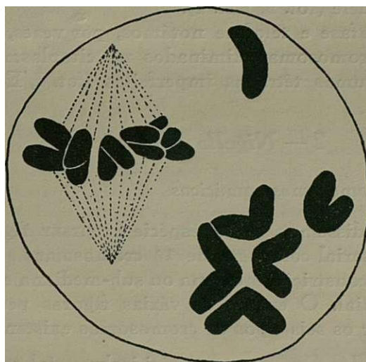
Fig. — N. damascena L. Metafase II mostrando uma das placas com os seis cromosomas bem orientados no fuso e a outra com cinco cromosomas no plano equatorial e uma fora dele. Carnoy; Carmim-acético. X 2.000.
