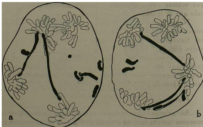
Fig. 7. — Ranunculus Ficaria L. (n.º 130). Anafases da segunda divisão vendo-se em a uma ponte persistente da primeira e uma da segunda, um fragmento e alguns univalentes em divisão, e em b uma ponte persistente da primeira divisão e duas formadas na segunda; à esquerda um univalente em divisão. Álcool acético;orceína acética. X 1100
