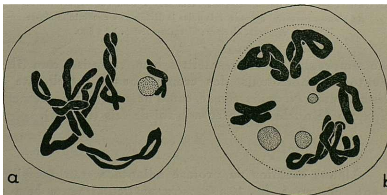
Fig. 10.— N. sativa L. a), Estádio da profase mostrando seis bivalentes e um nucléolo a que está ligado o bivalente constituído pelos cromosomas VI. b), Diacinese com seis bivalentes e tres nucléolos. Carnoy; Carmim-acético. X 1.600.
