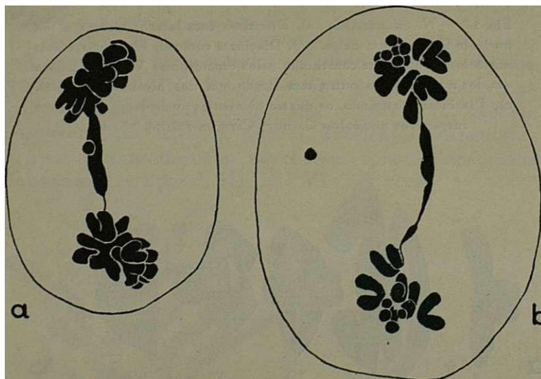
Fig. 19__- N. ciliaris DC. a) e b), Telofases I mostrando ponte provida de fragmento . Carnoy; Carmím-acético. a X 1.800. X 1.600.
