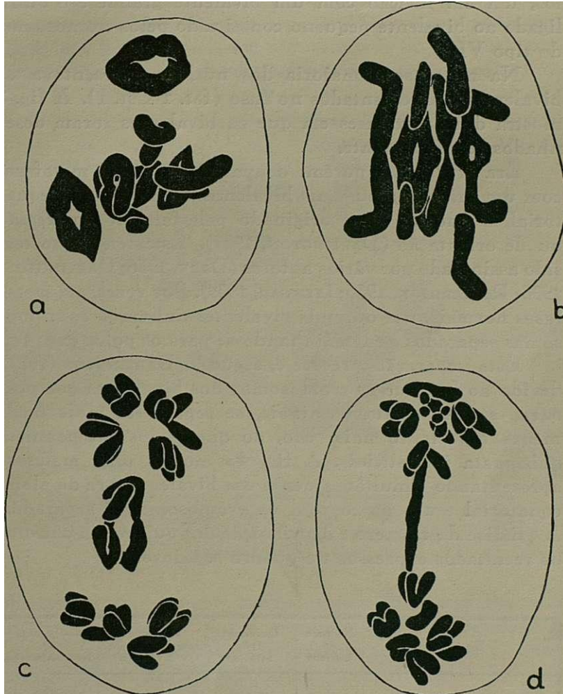
Fía. 4.— N. damascena L. a), Metaíase I mostrando um bivalente situado na região de um dos polos e o outro já dividido. b), Metafase I mostrando dois bivalentes já separados e encaminhando-se para os polos. c), Anafase I mostrando no plano equatorial dois bivalentes que se não dividiram. d), Anafase I apresentando dois cromosomas homólogos ainda não separados completamente. Carnoy; Carmim-acético. X 2.000.
