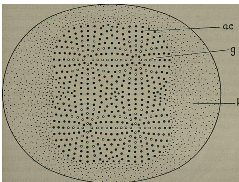
Fig. 7 — Un chromomère en train de se diviser (séparation des deux régions actives en quatre faisceaux). Représentation schématique. ac — acide nucléique propre du gènonema; g — genonema; k — kalymma.
