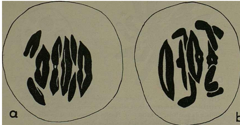
Fig. 11.— N. sativa L. a) e b), Metafases I com os seis Bivalentes no plano equatorial estando dois deles já divididos e encaminhando-se para os polos. Carnoy; Carmin-acético. X 1.600.
