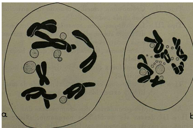
Fig. 26. — N. gallica Jord. a), Diacinese com seis bivalentes e seis «nucléolos». Carnoy; Carmim-acético. X 2.700. b), Diacinese apresentando vários corpos semelhantes a nucléolos. Carnoy; Carmim-acético. X 1.600.
