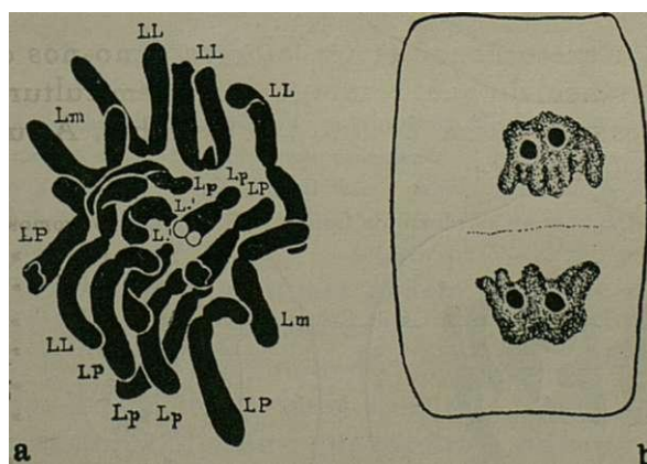
Fig. 1. — Ranunculus Ficaria L. (n.º 151). a, Placa equatorial numa célula do vértice vegetativo da raiz. Nav.-viol. gén. X 2330. b, Telofase mostrando 2 nucléolos em cada grupo polar. Flemming; safranina verde luz. \times 1800 .
