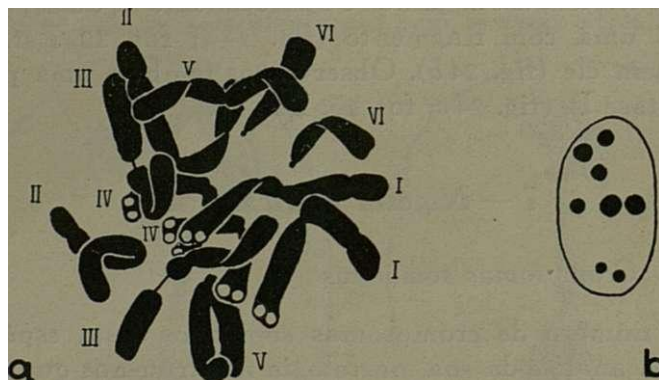
Fig. 25. — N. gallica Jord. a), Placa ecuatorial numa célula do meristema radicular mostrando os seis tipos de cromosomas. Navachine; Violeta de génciann. X 2.700. b), Núcleo de uma célula do meristema radicular; vêem-se oito nucléolos. Altmann. X 2.700.
