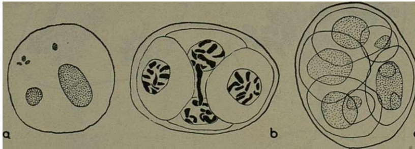
Fig. 21. — N. ciliaris DC. a), Telofose II com os grupos polares de tamanhos muito diferentes. b), Ponte que persistiu até à formação da tétrada. c), «Tétrada» anómala. Carnoy; Carmim-acético. X 900.
