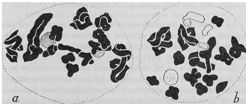
Fig. 3 — O. Eigii Feinbr. Diacinèses dans des cellules des grains de pollen, a , 4 IV-f 10 II; b , 2 IV-f 1 III-f-11 II-f-3 I. Alcool acétique-carmin acétique. X 1.200.
