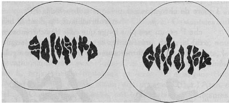
Fig. 2 — O. paterfamilias Godr. Métaphases I dans les cellules-mères des grains de pollen. 9 bivalents. Alcool acétique-carmin acétique. X 900.
