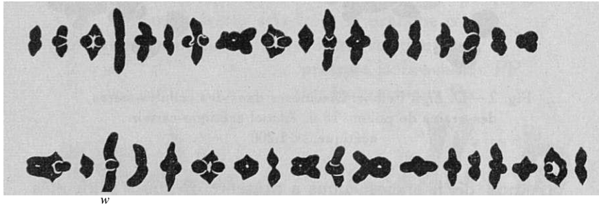
Fig. 4 — O. Eigii Feinbr. Les 18 bivalents de deux métaphases dessinés séparément. Alcool acétique-carmin acétique. X 1.200.
