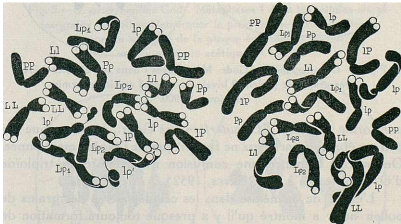
Fig. 1 — O. paterfamilias Godr. Métaphases dans des cellules du méristème racinaire. Navachine-violet de gentiane. X 3.200.
