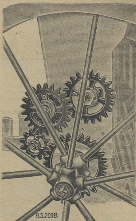
Fig. 38 — Posição da engrenagem para saída superior da semente
