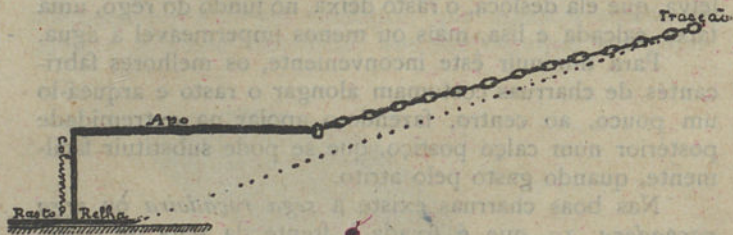
Fig. 6 — Linhas gerais da charrua
