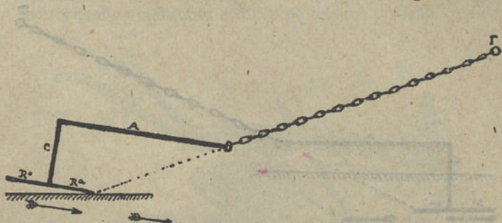
Fig. 7 — Linhas gerais da charrua. Posição que toma a charrua ao ser acionada; o bico da relha tende a ferrar-se na terra.
