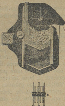
Fig. 29 — Distribuidor Schloer
