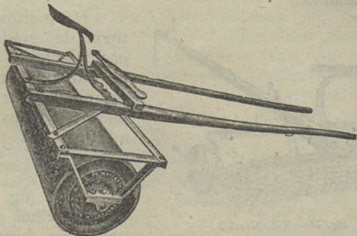
Fig. 22 — Rólo calcador
