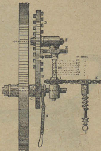
Fig. 41 — Regulador de distribuição Japy
