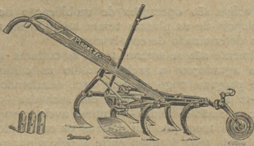
Fig. 25 — Sachador Planet
